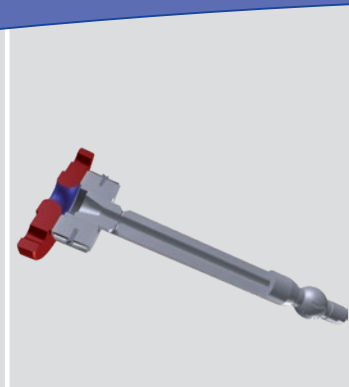
3: Schnitt durch das CIPPY-System mit Reinigungsdüsen im Einleitrohr
